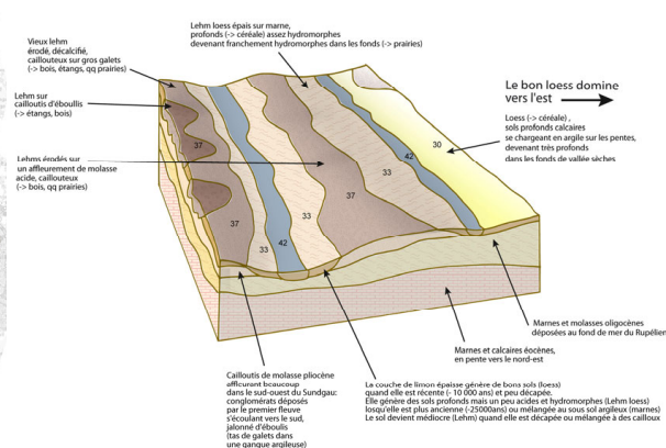
Sundgau bloc-diagramme roche et sol
