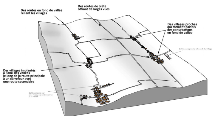
Sundgau bloc urba
